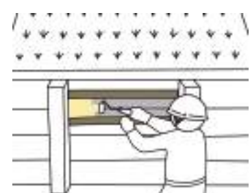
9. コーティング材を塗布します。(1回目塗布)
