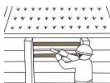
7. シール材をヘラで均します。
