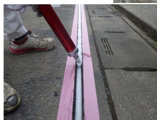
ロードセイバーシリコンシーラント注入
